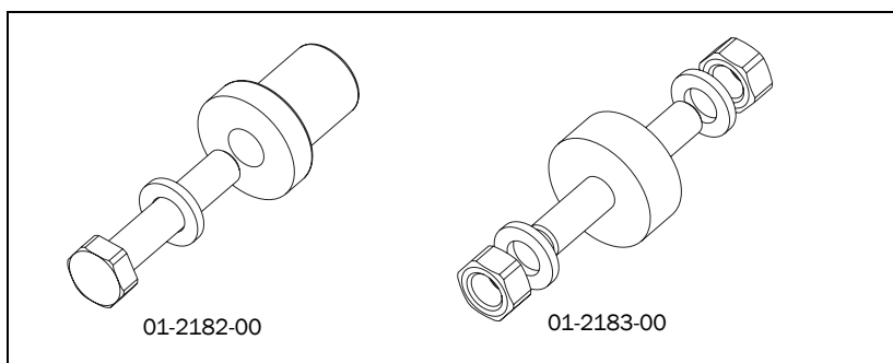
Afb. 8 Montagetoebehoren met trillingsdemping voor de motor
