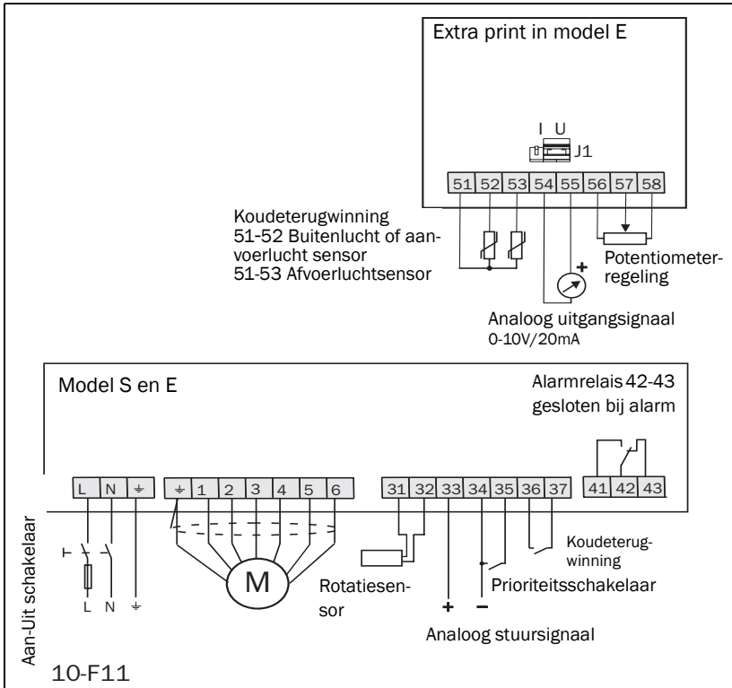
Fig. 5 Bedradingschema
