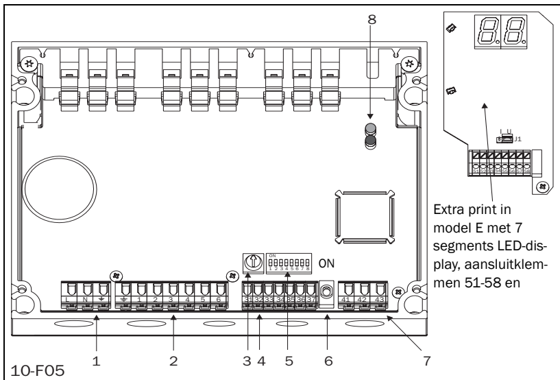
Fig. 4 Positie van aansluitklemmen, enz.
