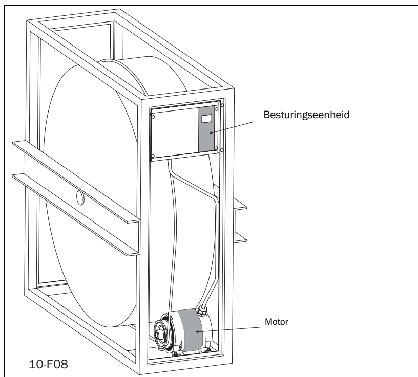
Fig. 1 Rotor met aandrijfsysteem
