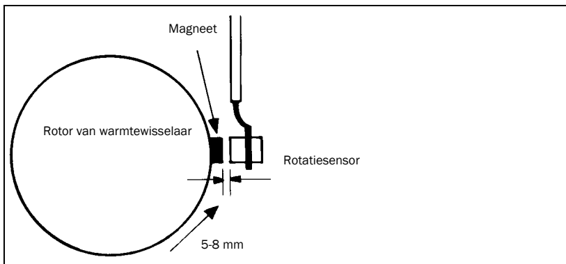
Fig. 2 Installatie van rotatiesensor
