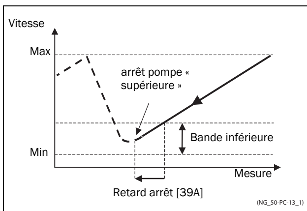
Fig. 114 Bande inférieure.
