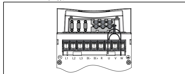
Fig. 22 Emotron VFX Modèles 48-060 à 48-105 (taille de châssis D2), Modèles 69-033 à 69-058 (taille de châssis D2(69)), vue arrière.
