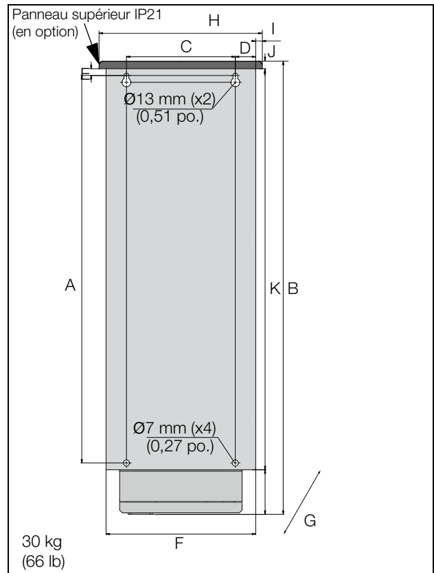
Fig. 22 Emotron VFX Modèles 48-060 à 48-105 (taille de châssis D2), Modèles 69-033 à 69-058 (taille de châssis D2(69)), vue arrière.
