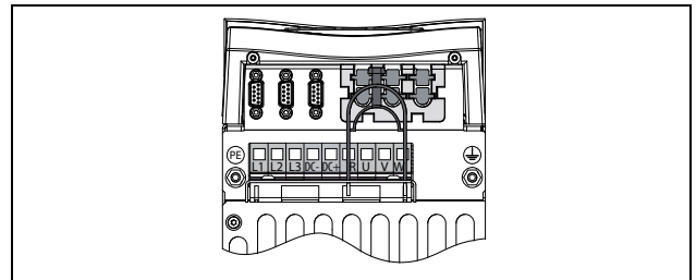
Fig. 17 Vue inférieure Emotron VFX Modèles 48-025 à 48-058 (format de châssis C2), Modèles 69-002 à 69-025 (format de châssis C2(69)), avec interface de câble pour l'alimentation, le moteur, CC+/CC-, la résistance de freinage et le contrôle.
