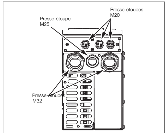
Fig. 19 Interface de câblage pour l'alimentation, le moteur et la communication, Emotron VFX Modèles 69-002 à 025 (format de châssis C69).
