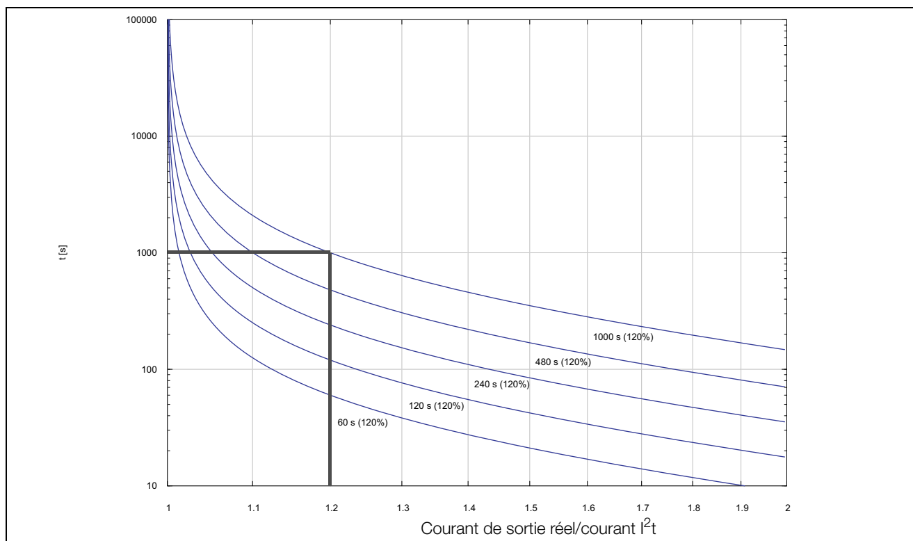
Fig. 93 Fonction I 2 t
