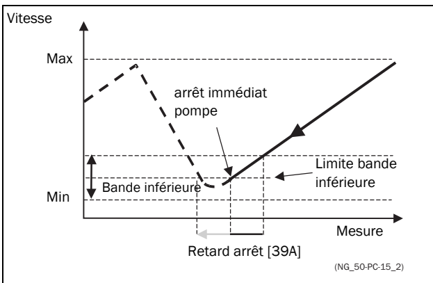
Fig. 116 Limite bande inférieure
