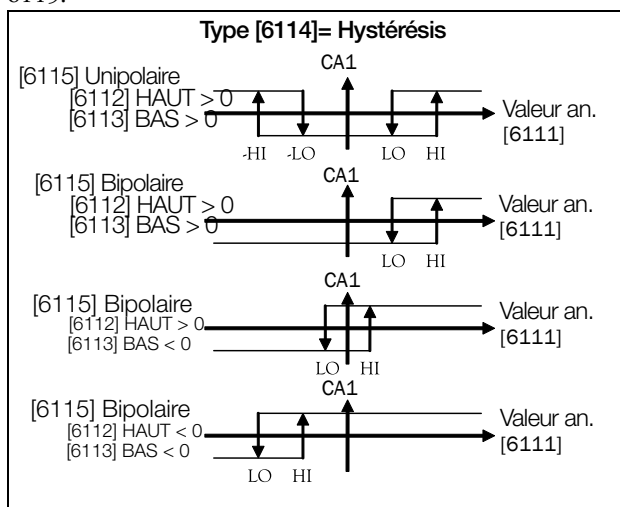
Fig. 134 Principe de fonctionnement des caractéristiques de comparateur pour « Type [6114] = Hystérésis » et « Polaire [6115] ».
