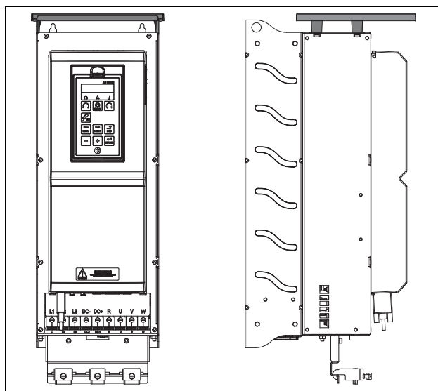
Fig. 159 Panneau supérieur en option monté sur le châssis de taille D2
