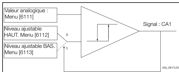
Fig. 130 Comparateur analogique de type Hystérésis
