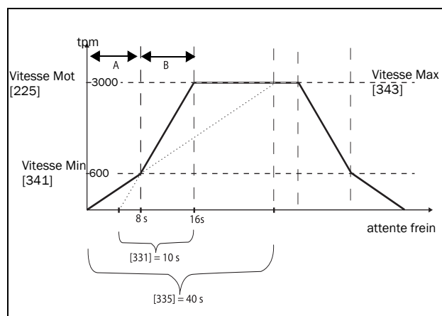
Fig. 98 Exemple de calcul des temps d'accélération (graphiques non proportionnels).
