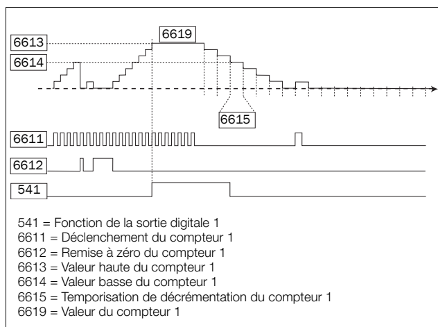
Fig. 141 Compteurs, principe de fonctionnement.
