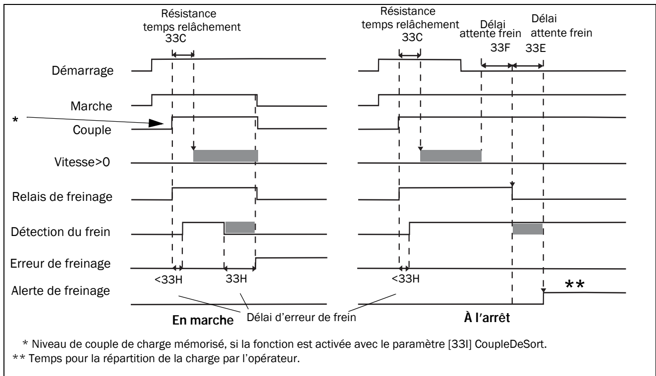
Fig. 102 Principe d'opération de freinage en cas de problème en marche et à l'arrêt.
