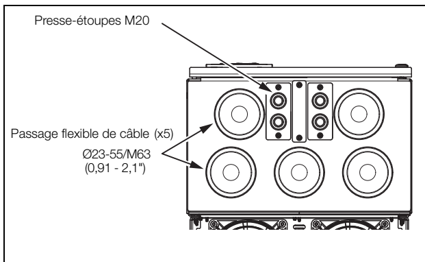
Fig. 32 Interface de câblage pour alimentation, moteur, CC+/CC-, résistance de freinage et communication, Emotron VFX Modèle 48-365-54 (taille de châssis FA).
