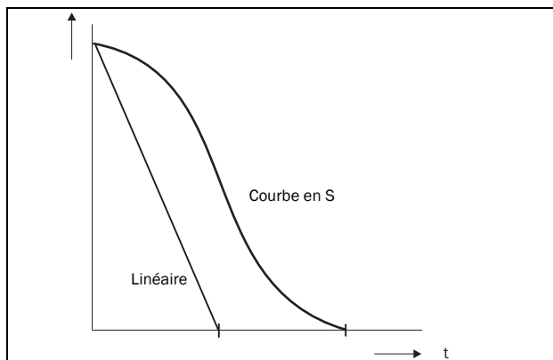
Fig. 100 Forme de la rampe de décélération
