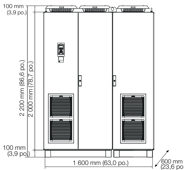
Emotron VFX48 : Modèles 1710 à 1820 (taille de châssis H5)
