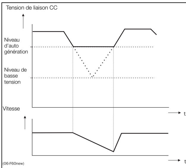
Fig. 123 Auto génération basse tension
