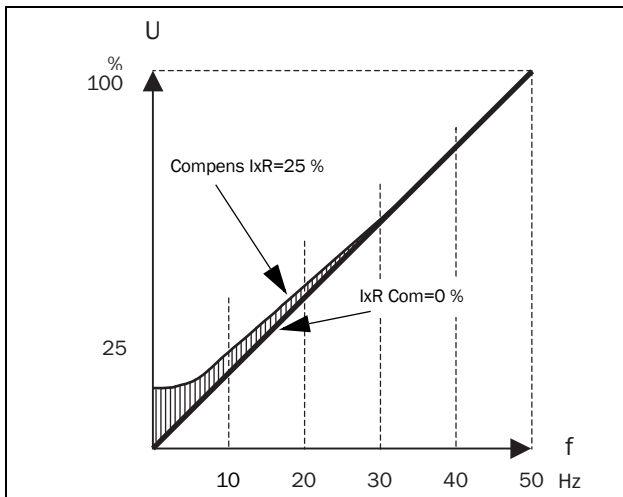
Fig. 106 Comp IxR sur une courbe linéaire V/Hz.
