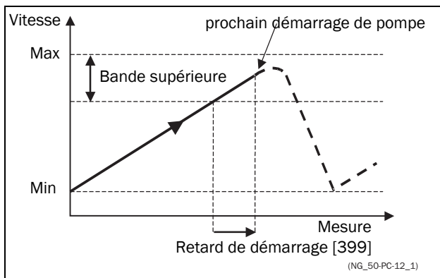
Fig. 113 Bande supérieure.
