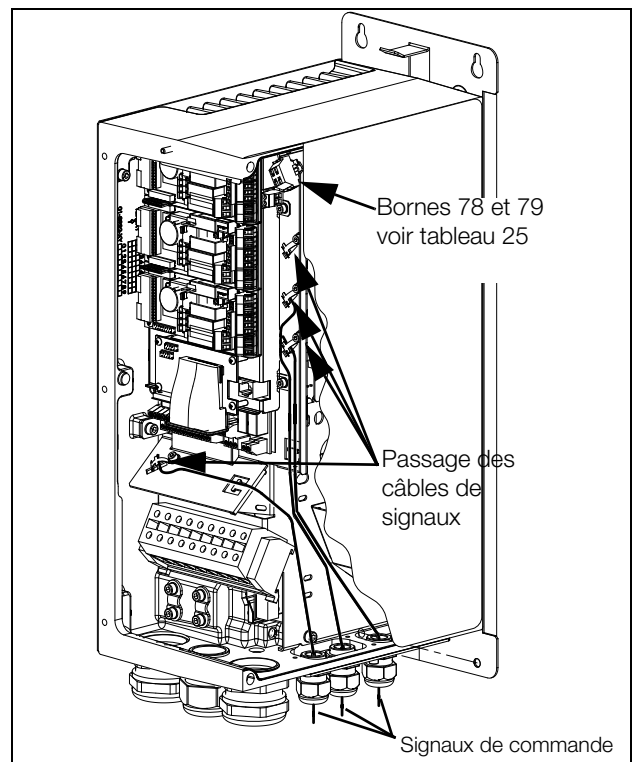
Fig. 65 Branchement des signaux de commande, VFX modèles 026 à 046, taille de châssis C.
