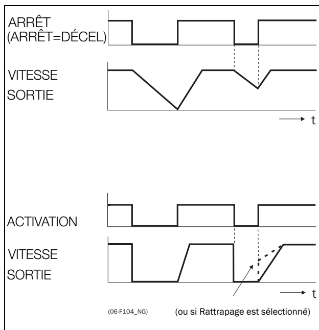
Fig. 77 Fonctionnalité de l'entrée Arrêt et Activation.
