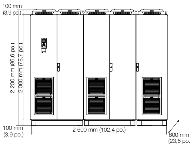
Emotron VFX48 : Modèle 2920 (taille de châssis H8) Emotron VFX69 : modèle 1K6 (taille de châssis M69)
