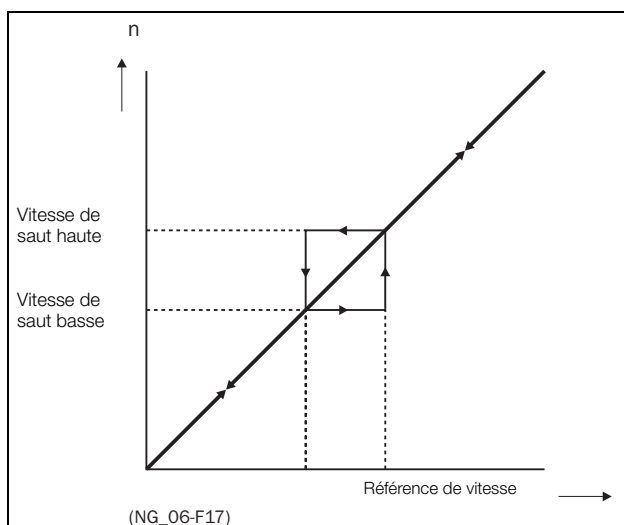
Fig. 104 Vitesse de saut
