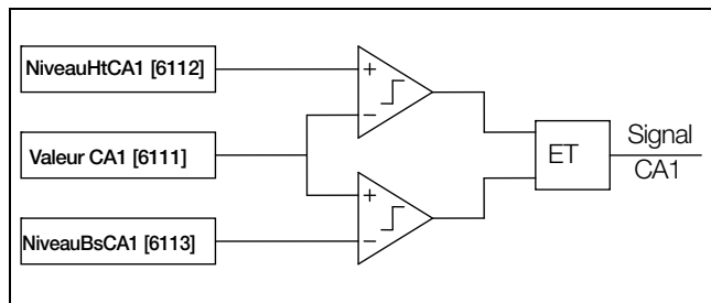
Fig. 131 Comparateur analogique de type « Créneau ».
