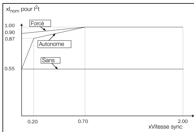
Fig. 92 Courbes I^2t .
