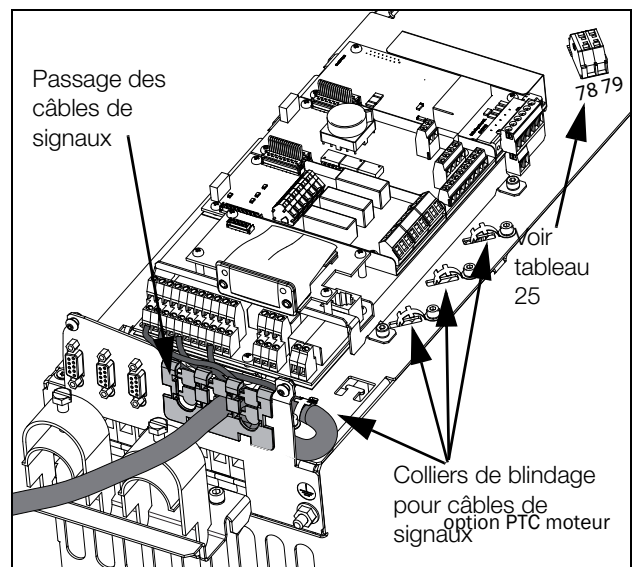
Fig. 66 Connexion des signaux de commande, VFX modèles 48-025 à 48-058 taille de châssis C2 et modèles 69-002 à 69-025 taille de châssis C2(69).
