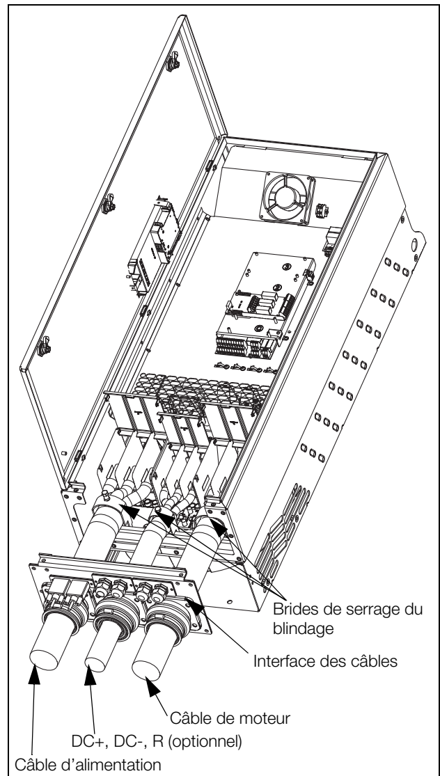
Fig. 50 Connexion des câbles d'alimentation et de moteur.
