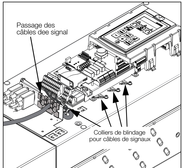
Fig. 70 Connexion des signaux de commande, VFX modèles 48-142 à 48-365 tailles de châssis E2, F2 et FA2 (schéma de principe).
