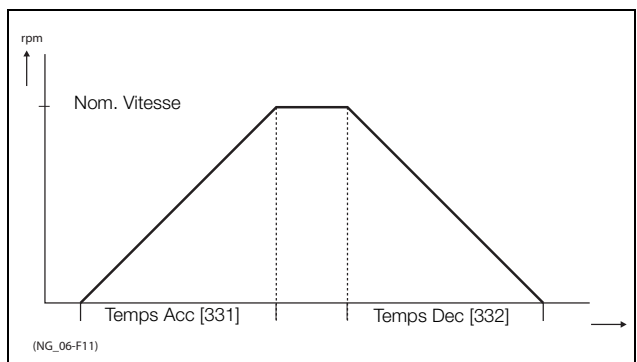
Fig. 97 Temps d'accélération et de décélération
