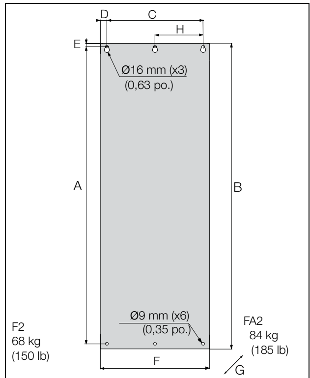
Fig. 30 Emotron VFX/ Modèles 48-205 à 48-293 (taille de châssis F2) et 48-365-20 (taille de châssis FA2).
