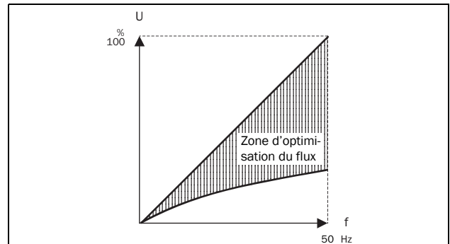
Fig. 107 Optimisation du flux
