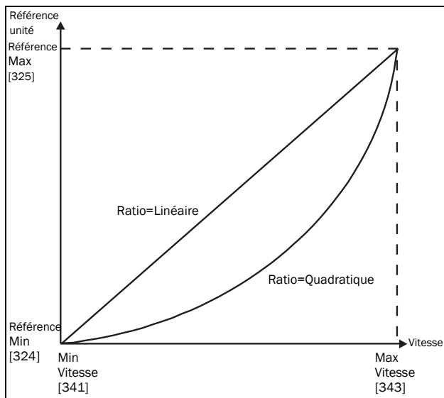
Fig. 94 Ratio.
