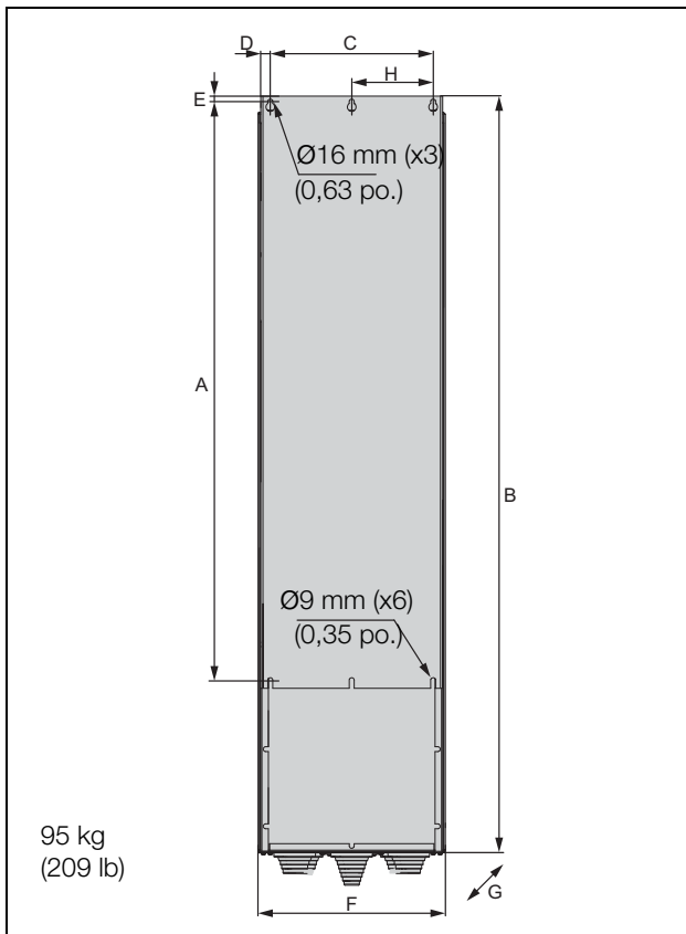
Fig. 31 Emotron VFX Modèles 48-365-54 (taille de châssis FA).
