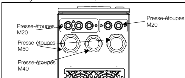
Fig. 20 Emotron VFX Modèles 48/52-061 à 074 (format de châssis D), Modèles 69-033 à 69-058, (format de châssis D69).
