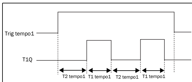
Fig. 138 Mode de temporisateur alternatif.
