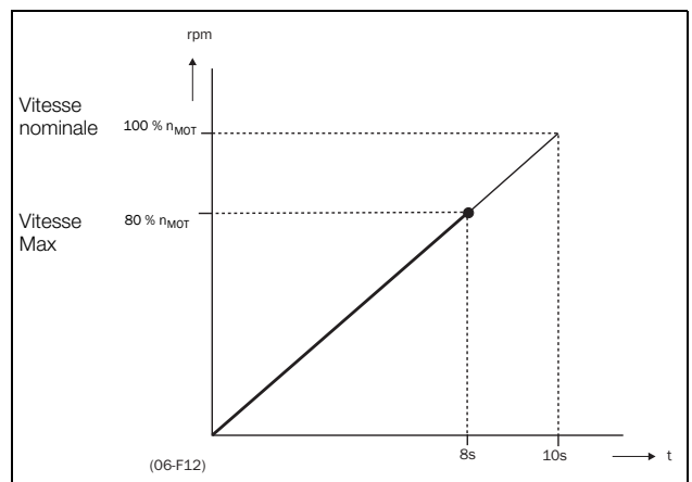
Fig. 96 Temps d'accélération et vitesse maximale
