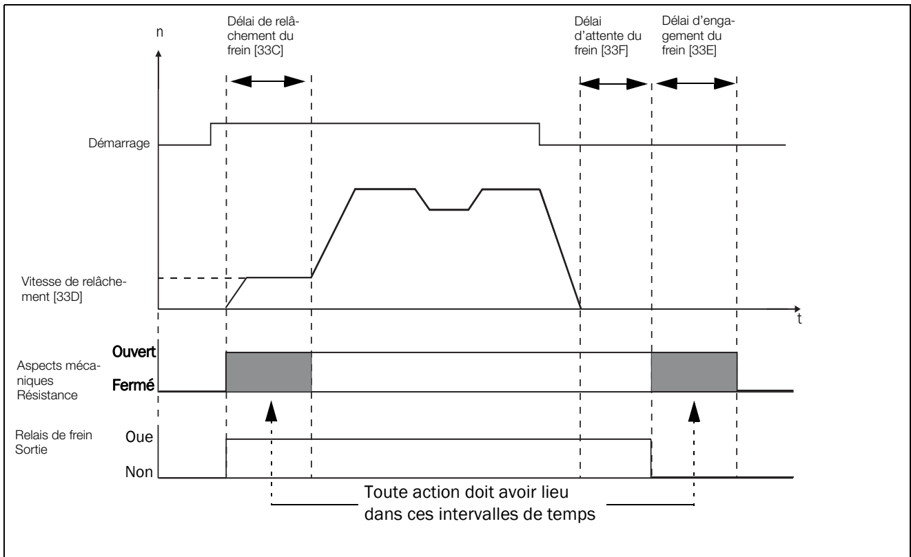
Fig. 101 Fonction de sortie de frein
