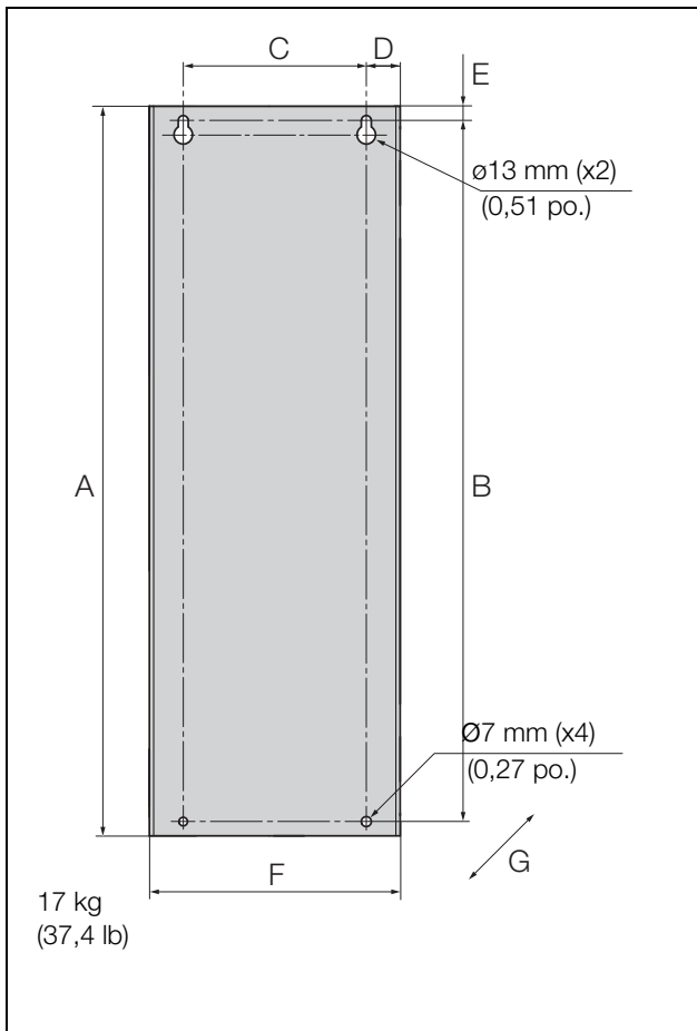
Fig. 18 Emotron VFX Modèles 69-002 à 025 (taille de châssis C69).
