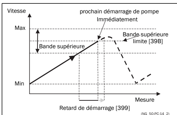
Fig. 115 Limite bande supérieure.
