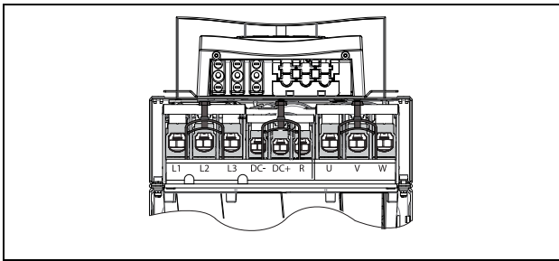
Fig. 29 Vue inférieure Emotron VFX/ Modèles 48-142 à 48-293 (format de châssis E2 et F2), avec interface de câble pour l'alimentation, le moteur, CC+/CC-, la résistance de freinage et le contrôle (schéma de principe).
