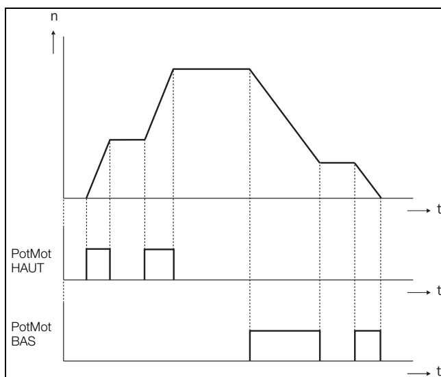
Fig. 108 Fonction PotMot.
