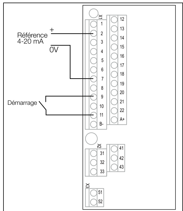
Fig. 74 Câblage
