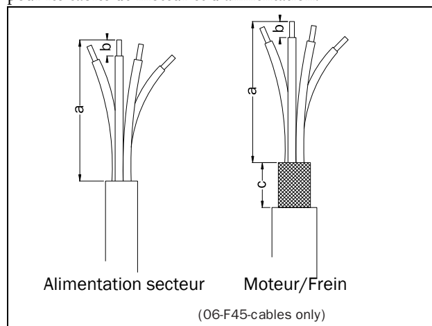
Fig. 59 Longueurs de câbles à dénuder
