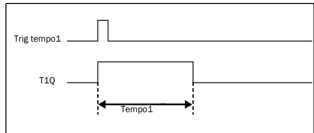
Fig. 139 Mode de temporisateur On-time
