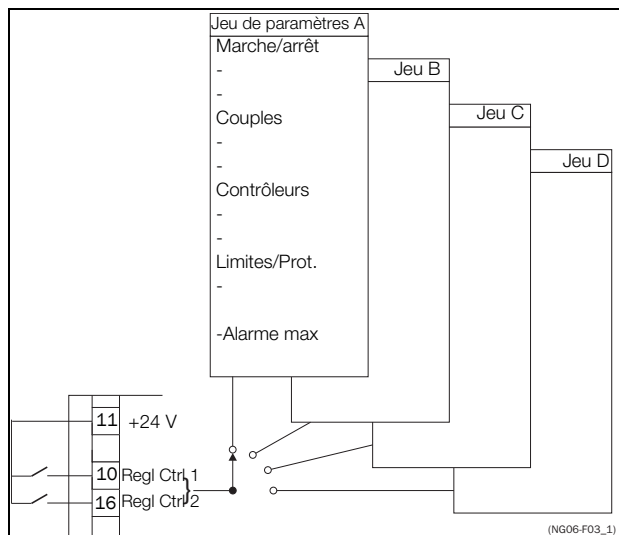
Fig. 75 Sélection des jeux de paramètres.
