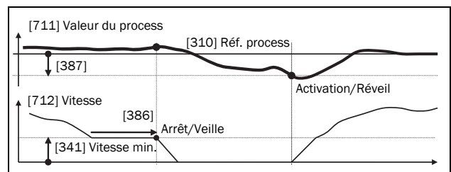
Fig. 110 Arrêt/veille PID avec PID normal
