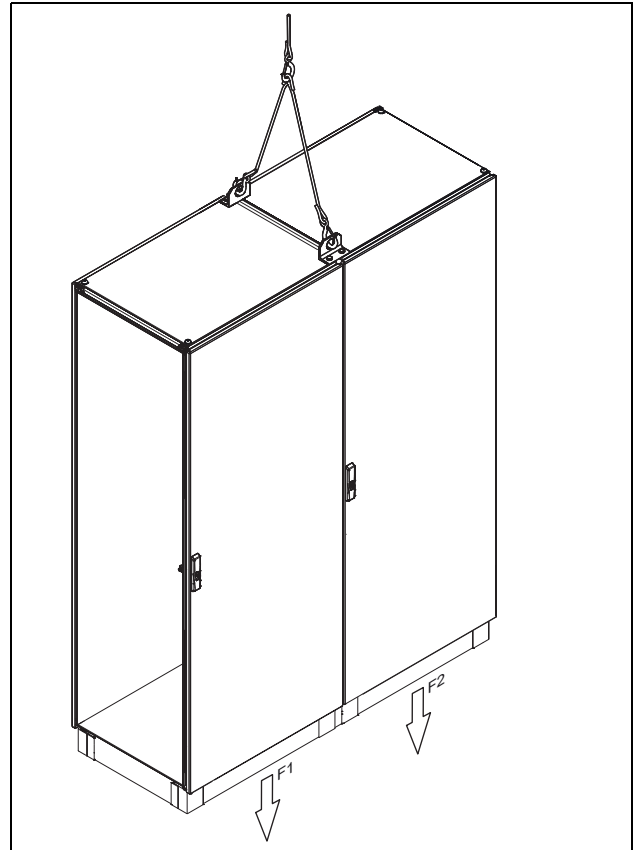
Fig. 6 Combinaison d'enceintes avec supports internes.
