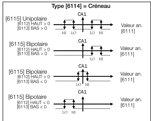
Fig. 135 Principe de fonctionnement des caractéristiques de comparateur pour Type [6114] = Créneau et Polaire [6115].
