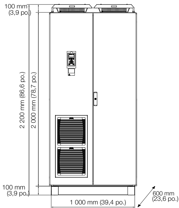
Emotron VFX48 : Modèles 810 à 1100 (tailles de châssis G3 et H3)
