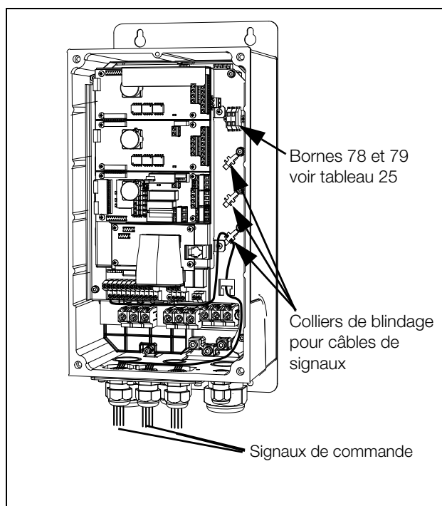
Fig. 64 Branchement des signaux de commande, VFX modèles 003 à 018, taille de châssis B.
