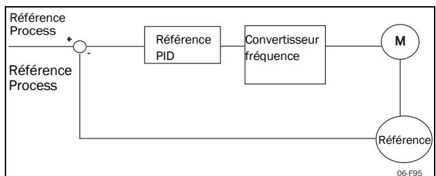
Fig. 109 Contrôle PID en boucle fermée
