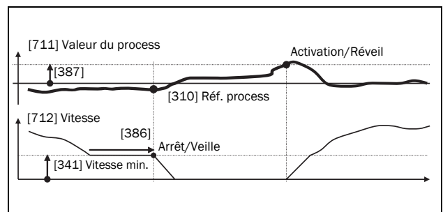
Fig. 111 Arrêt/veille PID avec PID inversé
