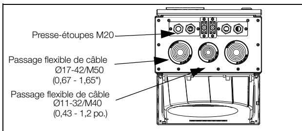
Fig. 25 Interface de câblage pour alimentation, moteur, CC+/CC-, résistance de freinage et communication, Emotron VFX Modèles 48-090 à 175 (format de châssis E).
