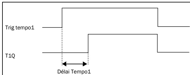
Fig. 137 Mode de temporisateur de délai.
